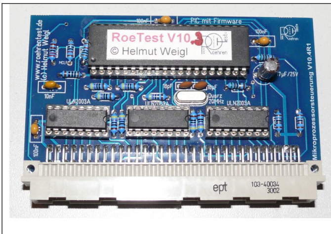
Mikroprozessorkarte RoeTest
