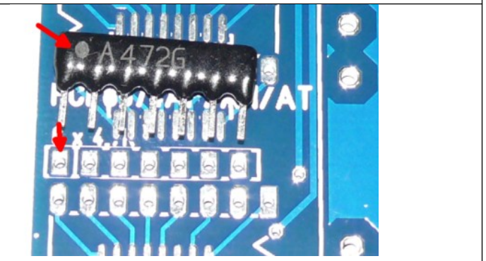
Widerstandsarray in richtige Richtung einbauen!
