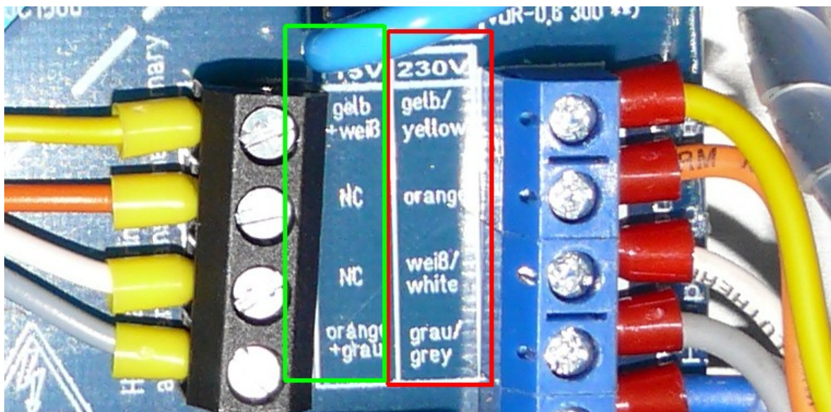
Das Bild zeigt den Anschluss der beiden Transformatoren bei 230V Netzspannung.
