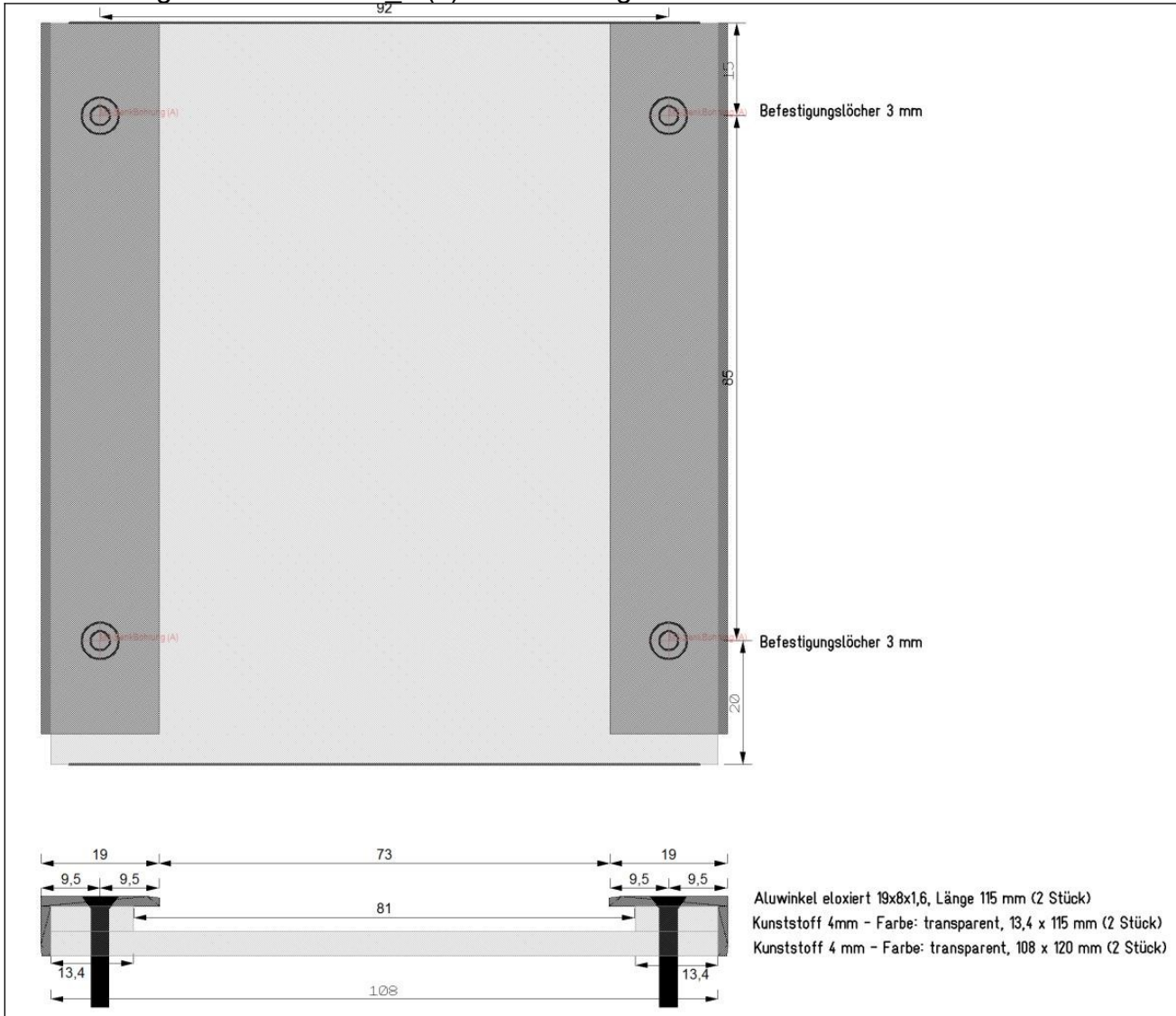
Zeichnung Fassungsboxhalter
